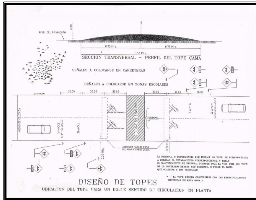
Fig. 1 Características y medidas obligatorias de un tope autorizado por la Secretaría de Movilidad.
